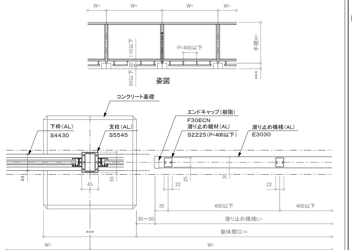
平面詳細図
