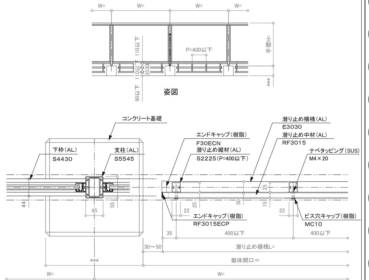
平面詳細図
