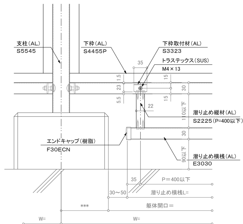
立面詳細図
