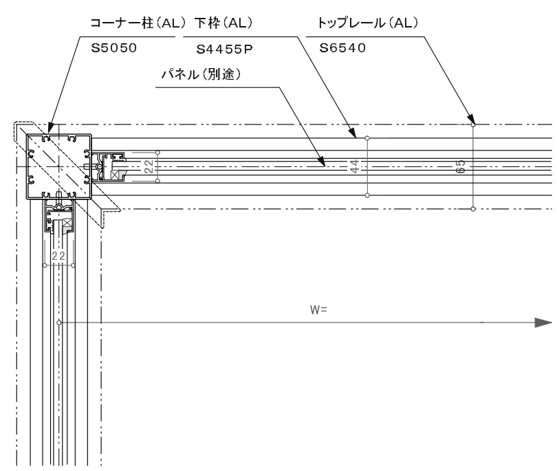
コーナー支柱納まり
