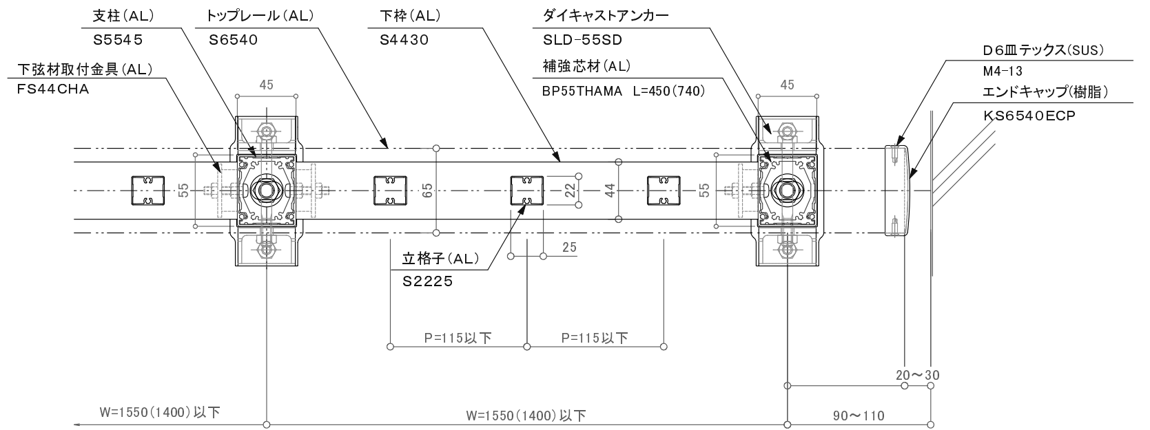
バルコニー用150型/KBS-2BDS(KBS-2BDSA)
