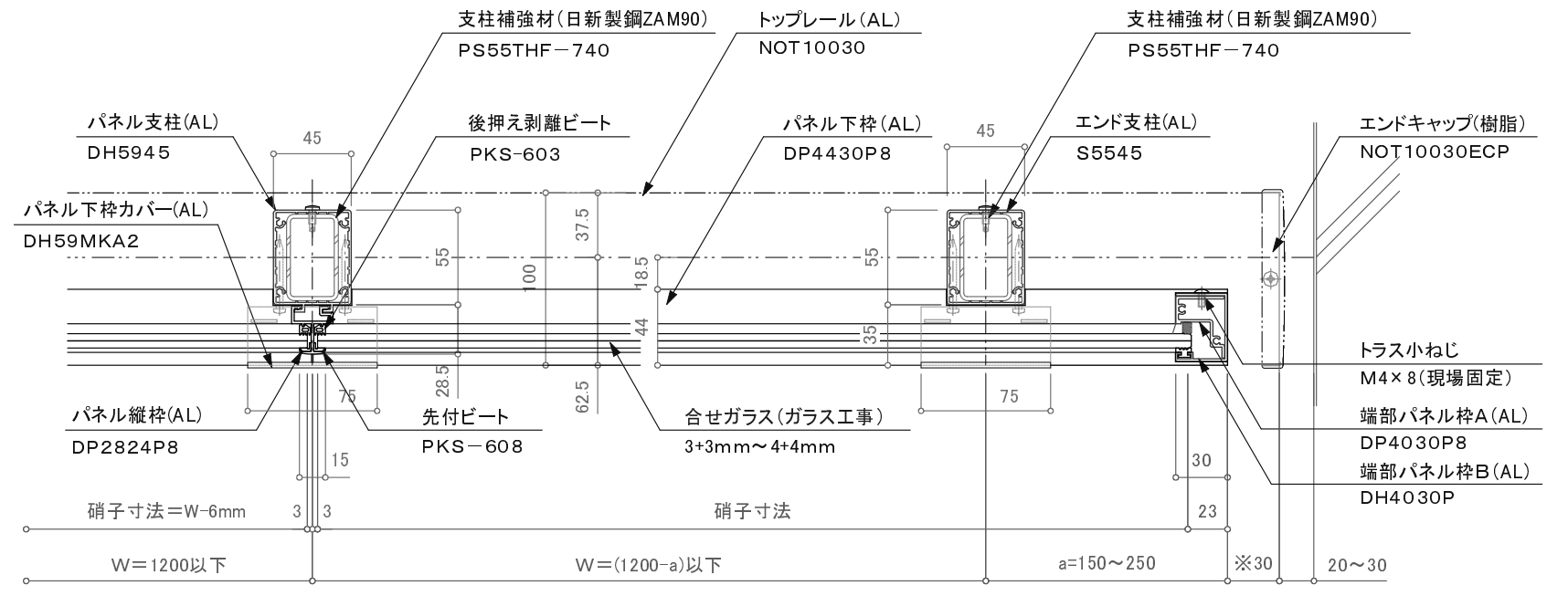
バルコニー用150型/FBS-SS-B
