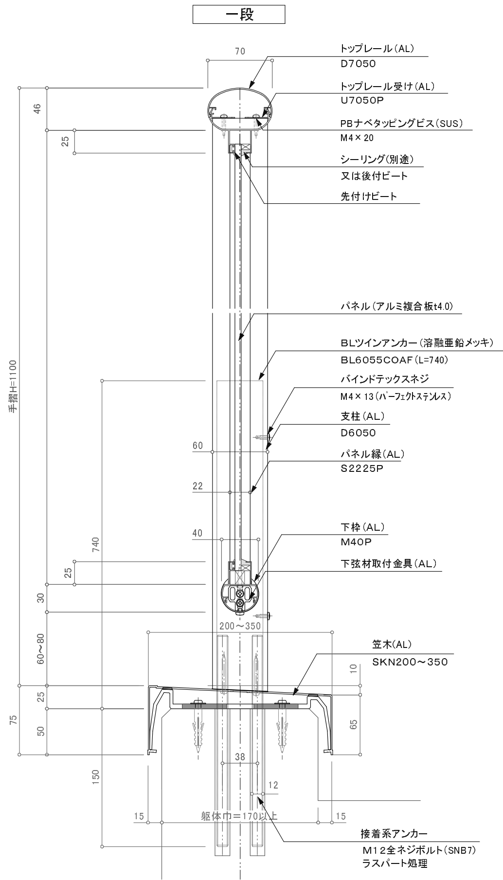
廊下用300型/DRK-2BW(一体型)
