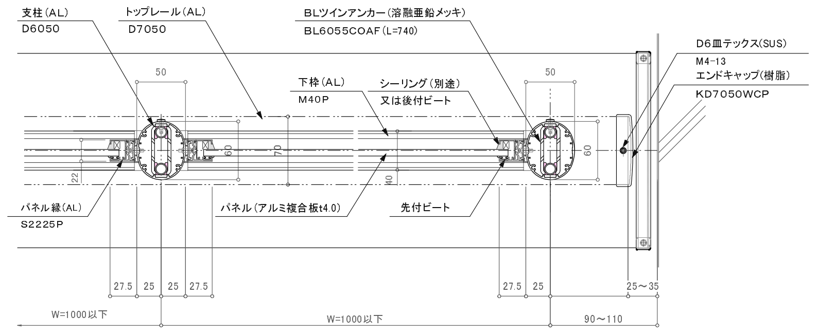
廊下用300型/DRK-2BW(一体型)
