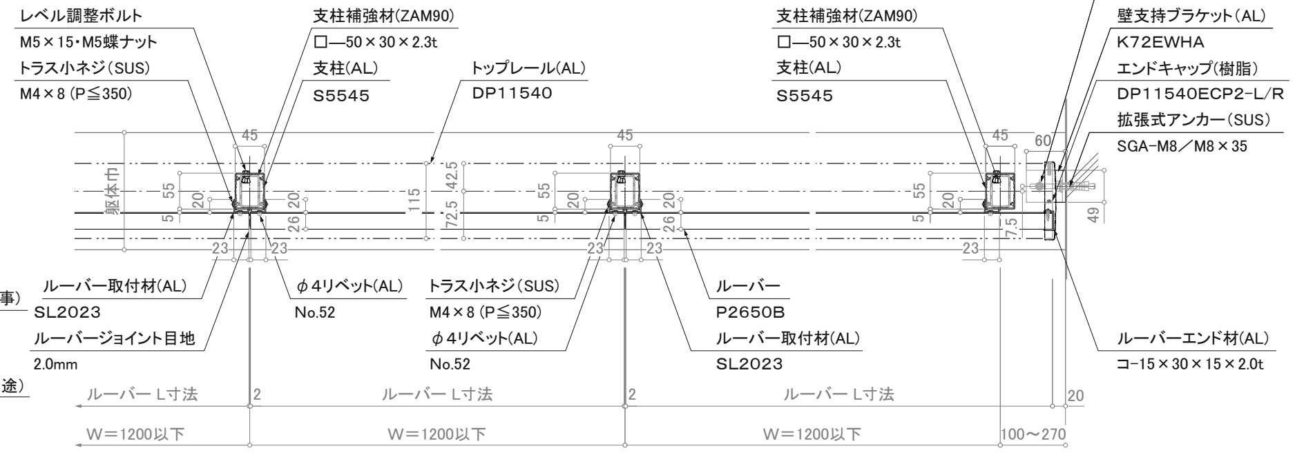
平面詳細図
