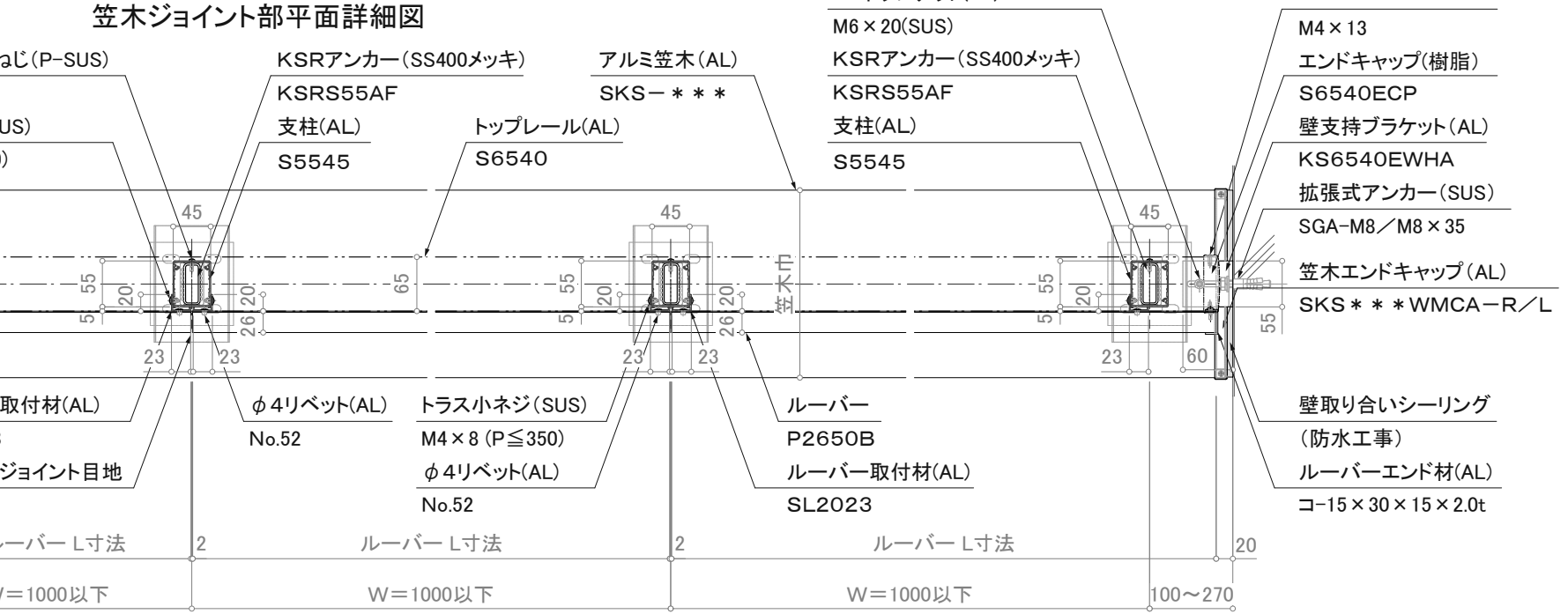
平面詳細図
