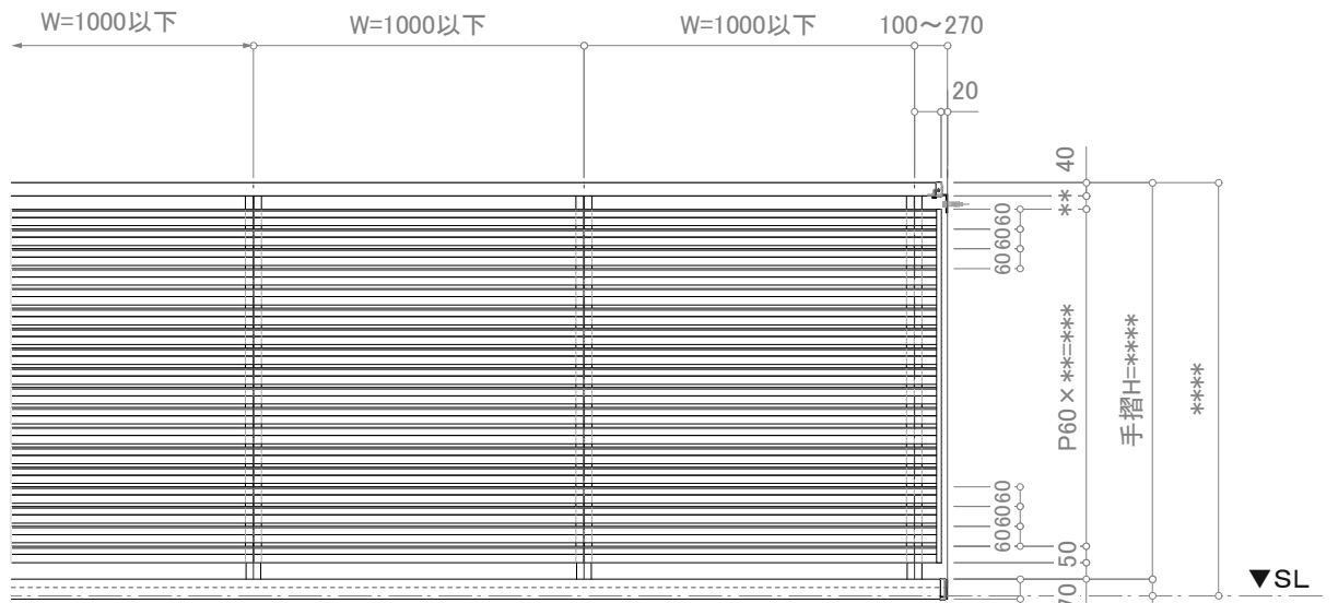
立面図
