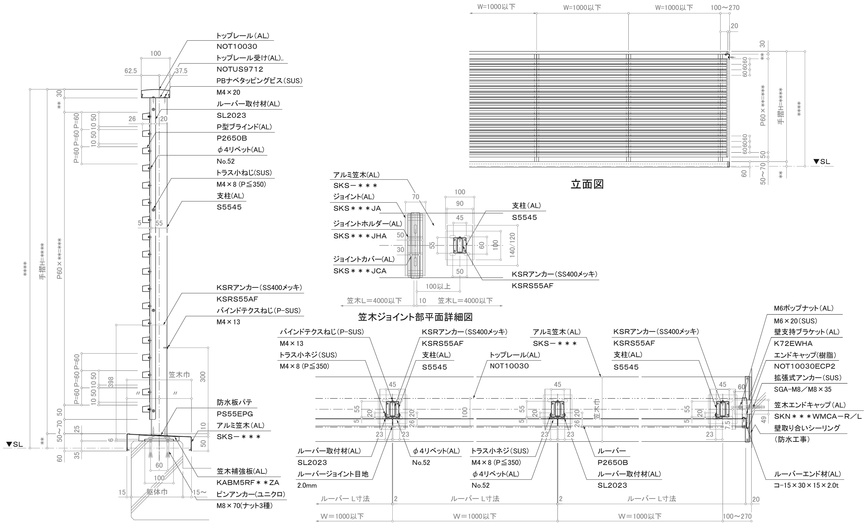
断面図
